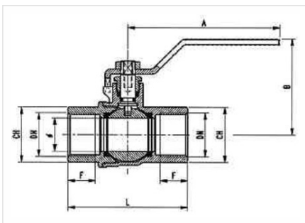
Robineti cu levier
