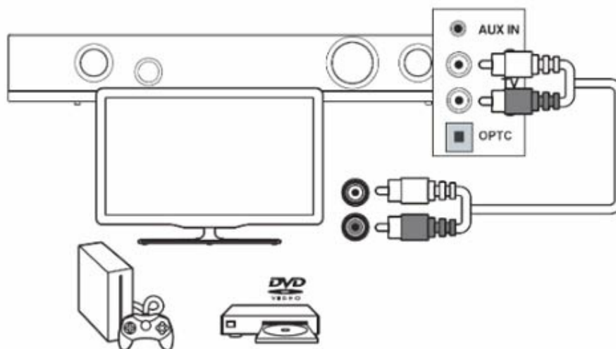
Anschluss-Beispiel per Audio-Cinch - Bildquelle Auna
