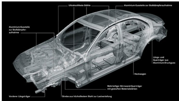
Leichtbau der neuen C-Klasse durch einen intelligenten Hybridverbund aus Stahl und Aluminium
